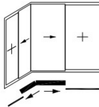
Bild: 12 Offene Ecke mit Außenflügel
