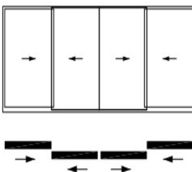
Bild: 8 Schiebe und Face to Face System
