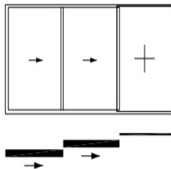
Bild: 6 Teleskoptür mit 2 Innenflügeln
