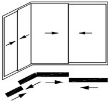
Bild 13 Offene Ecke mit Außenflügel und Slide - Slide System
