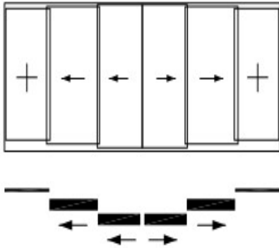
Bild: 11 Face to Face Slide - Schiebe und Teleskop Kombination
